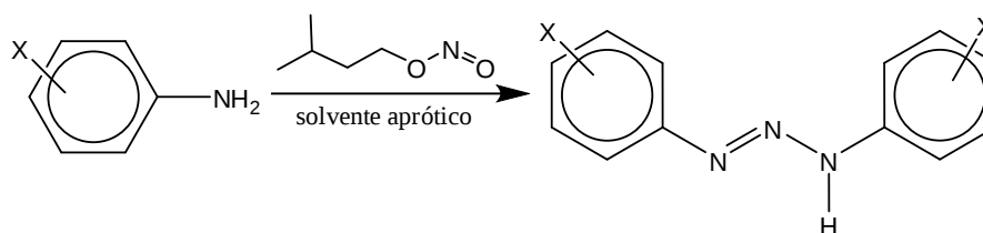
Figura 3 - Modelo Genérico das Reações com nitrito isoamílico
