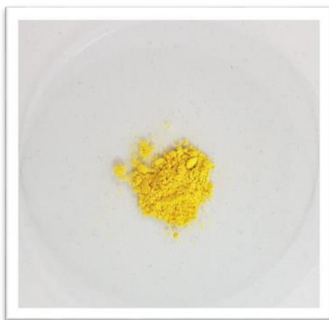
Figura 7 - Composto 1,3- bis (2-metoxi-5-nitrofenil)triazeno
