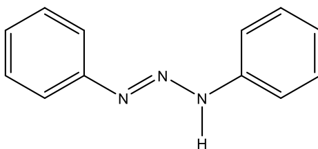
Figura 3. Representação estrutural do 1,3-bis(fenil)triazeno
