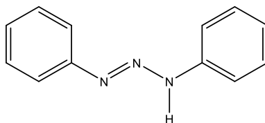
Figura 2 - Representação estrutural do 1,3-bis(fenil)triazeno
