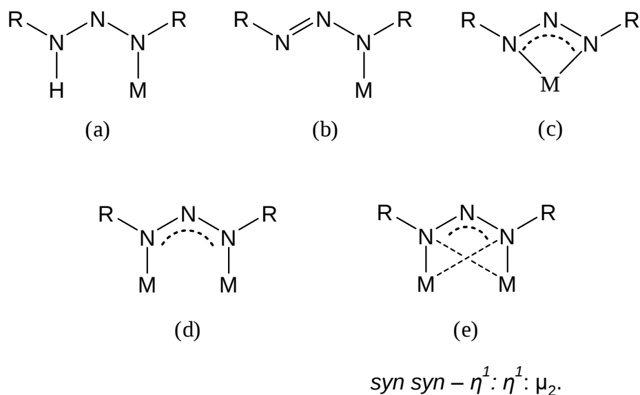
Figura 4. Principais modos de coordenação dos triazenos no estado sólido
