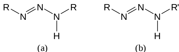
Figura 1 - Representação estrutural genérica de triazeno simétrico (a) e assimétrico (b)
