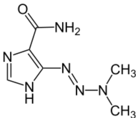
Figura 5. Representação da estrutura molecular do fármaco Dacarbazina
