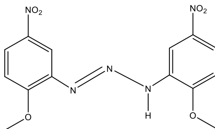
Figura 5 - Representação estrutural do 1,3-bis(2-metoxi-5-nitrofenil)triazeno
