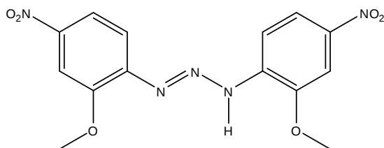
Figura 4 - Representação estrutural do 1,3-bis(2-metoxi-4-nitrofenil)triazeno
