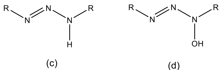
Figura 2. Representação estrutural genérica de triazeno (c) e hidroxitriazeno (d)
