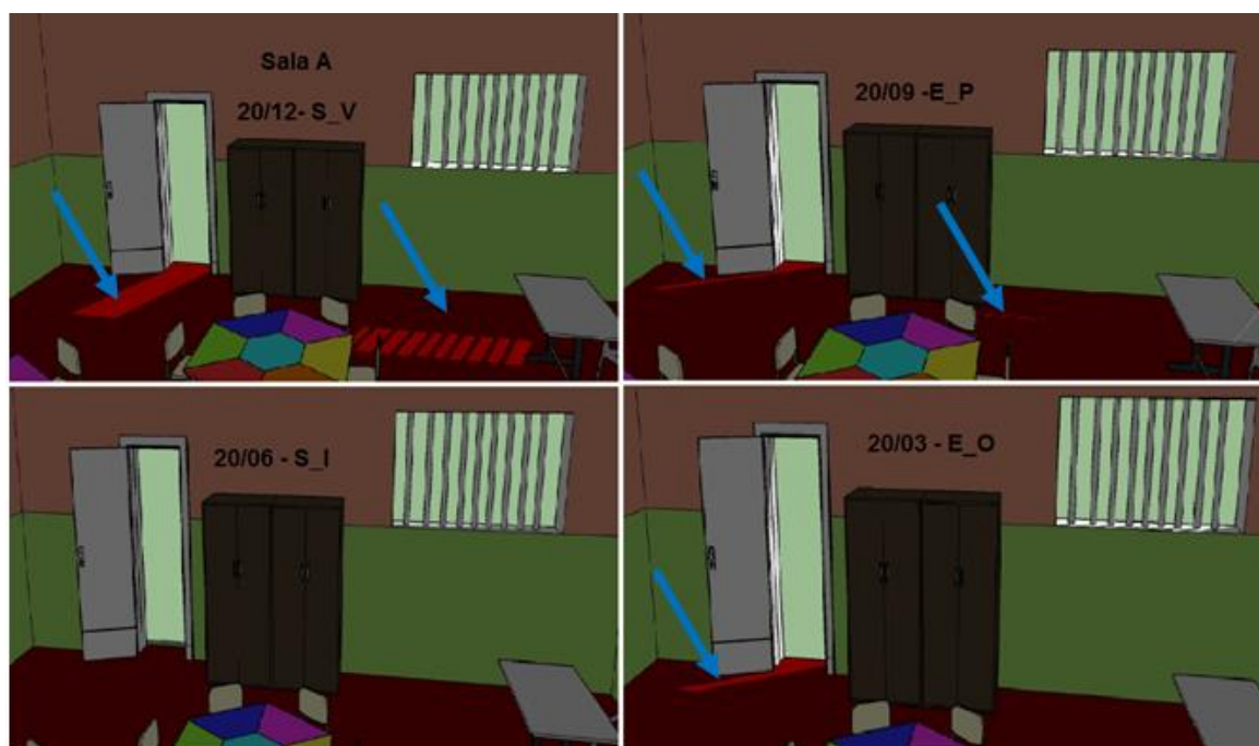
Figura 4 – Simulação de Incidência Solar às 15 horas na sala A. Fonte: Autor
