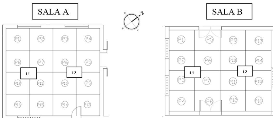
Figura 2 – Localização dos pontos de medição, salas A e B. L1 e L2 luminárias com duas lâmpadas Fluorescentes tubulares T8 de 32W
